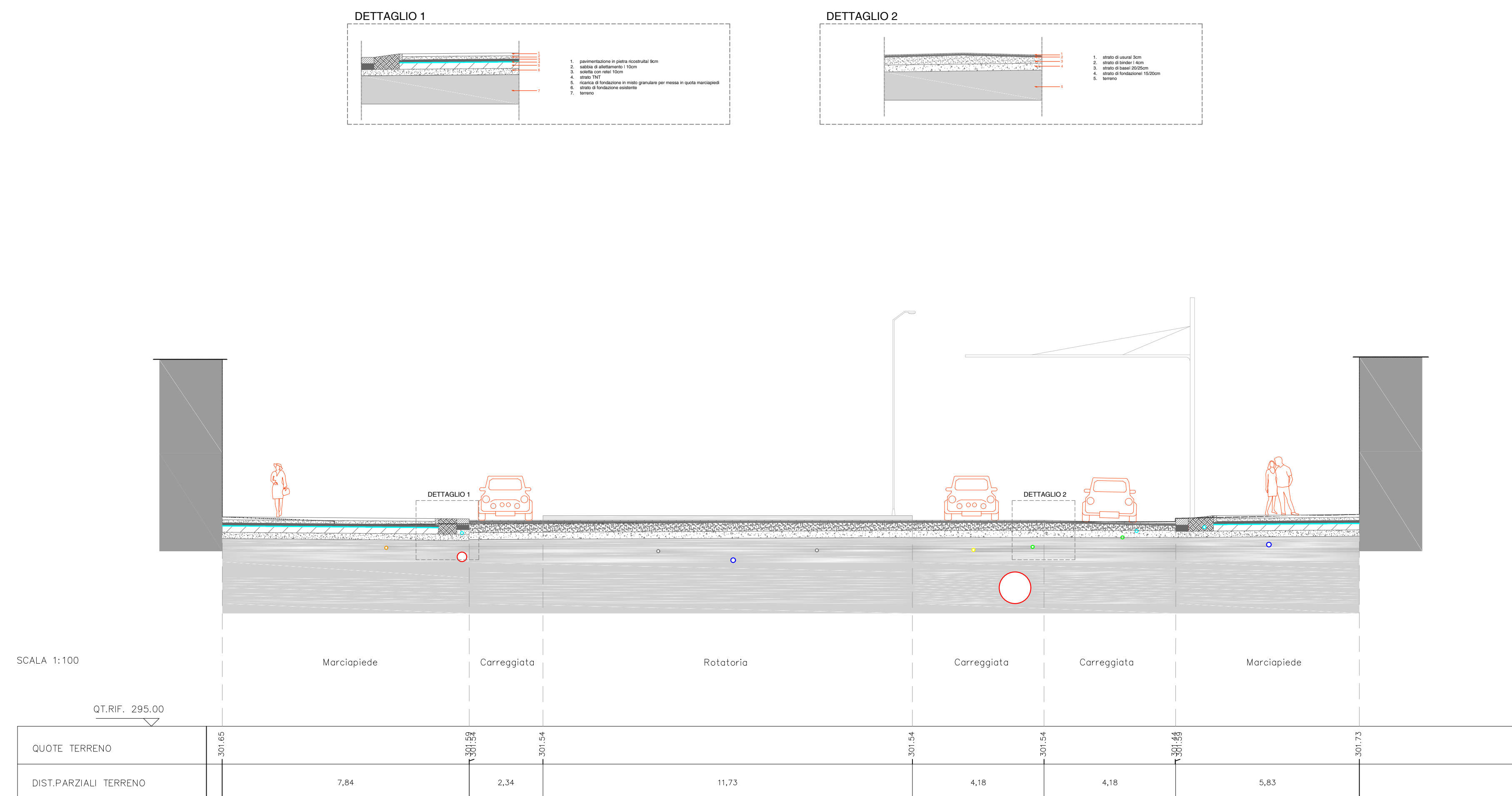
SEZIONE 1_distanza progressiva: 0.00 m
