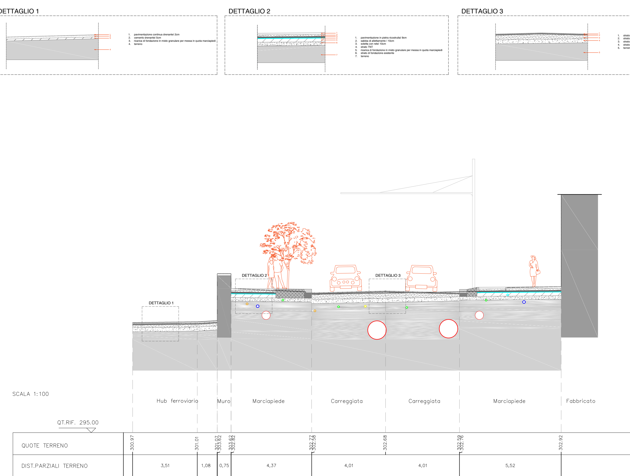
SEZIONE 6_distanza progressiva: 125.00
