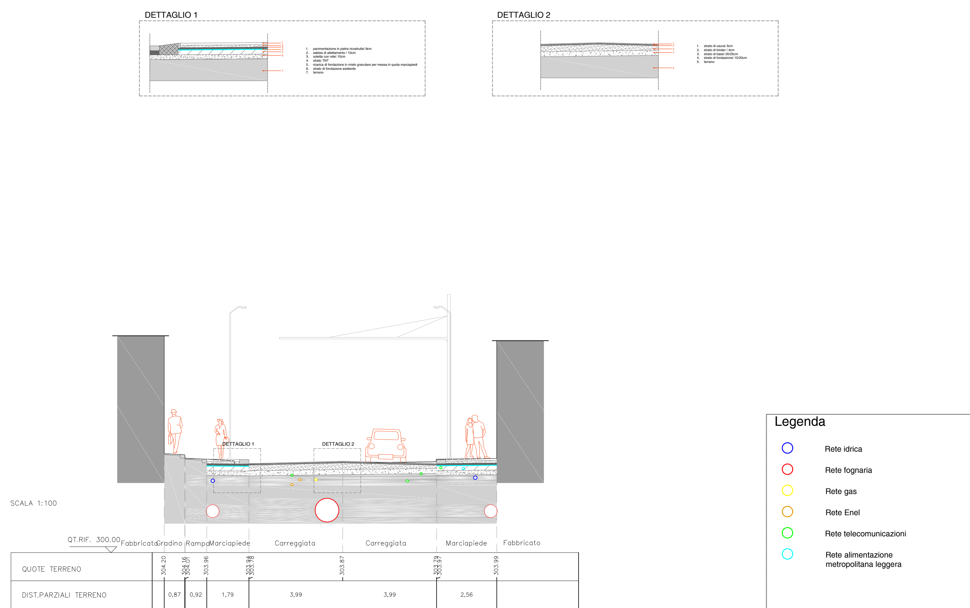
SEZIONE 15_distanza progressiva: 350.00
