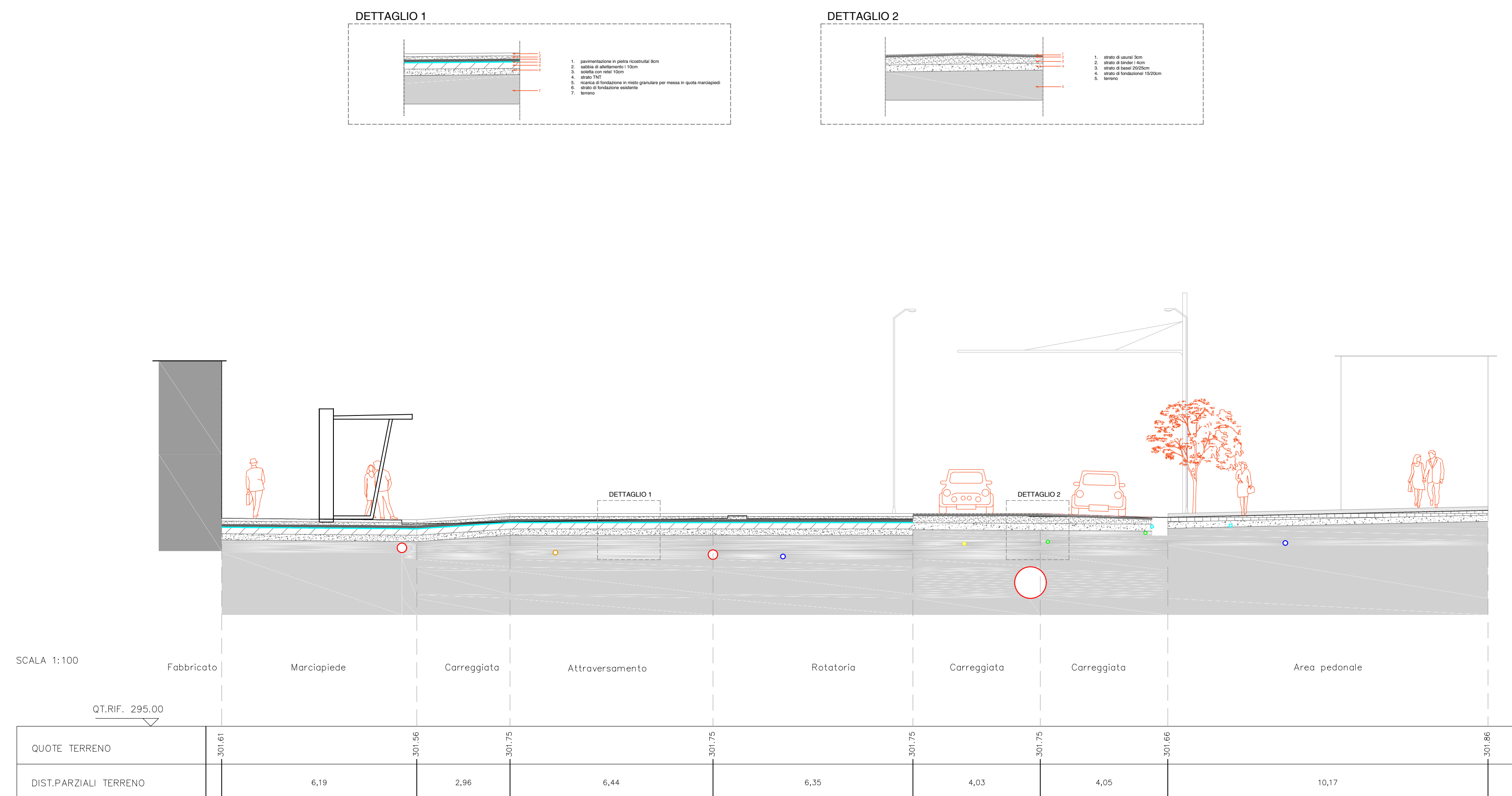
SEZIONE 2_distanza progressiva: 25.00 m
