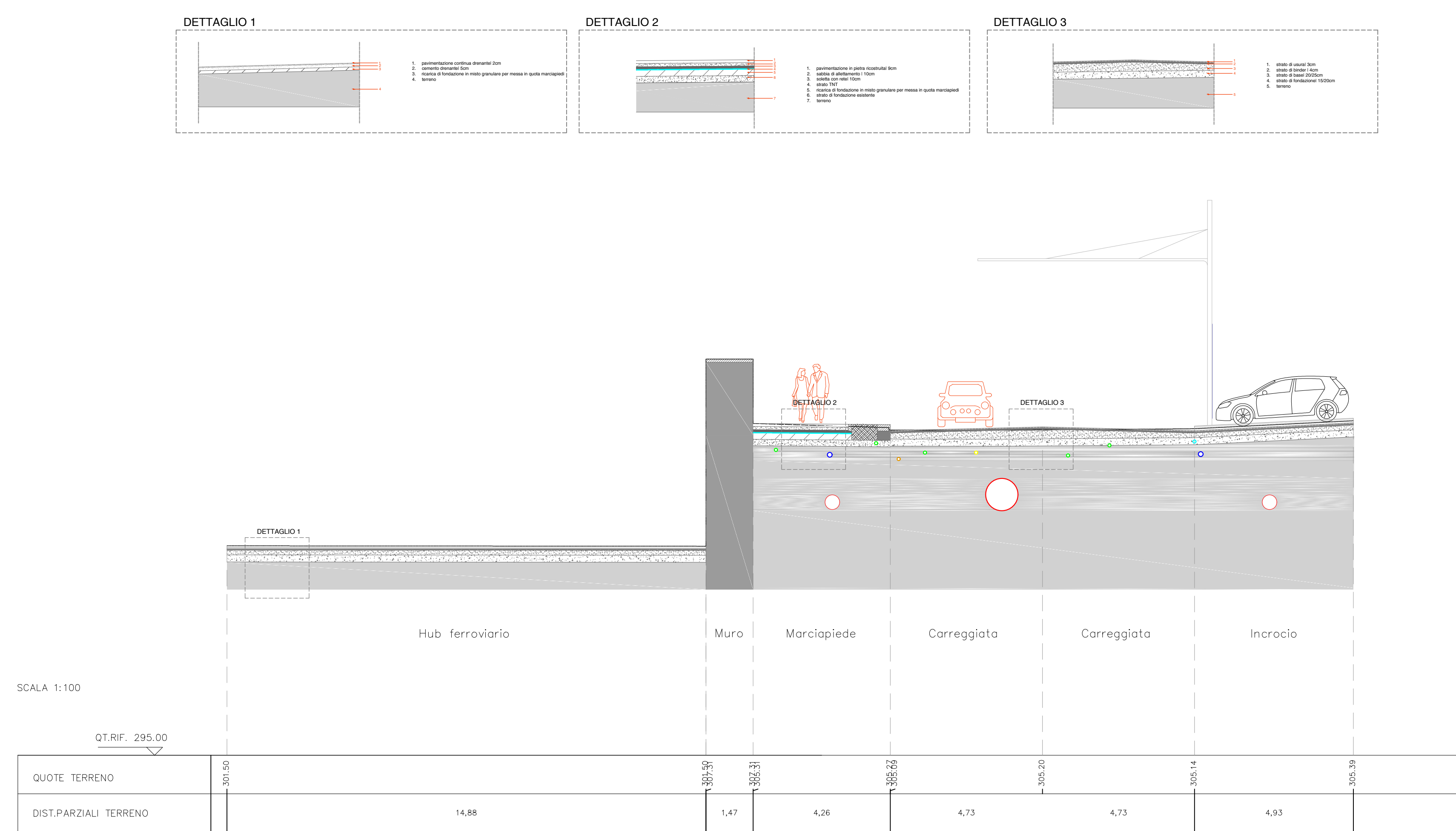
SEZIONE 10_distanza progressiva: 225.00
