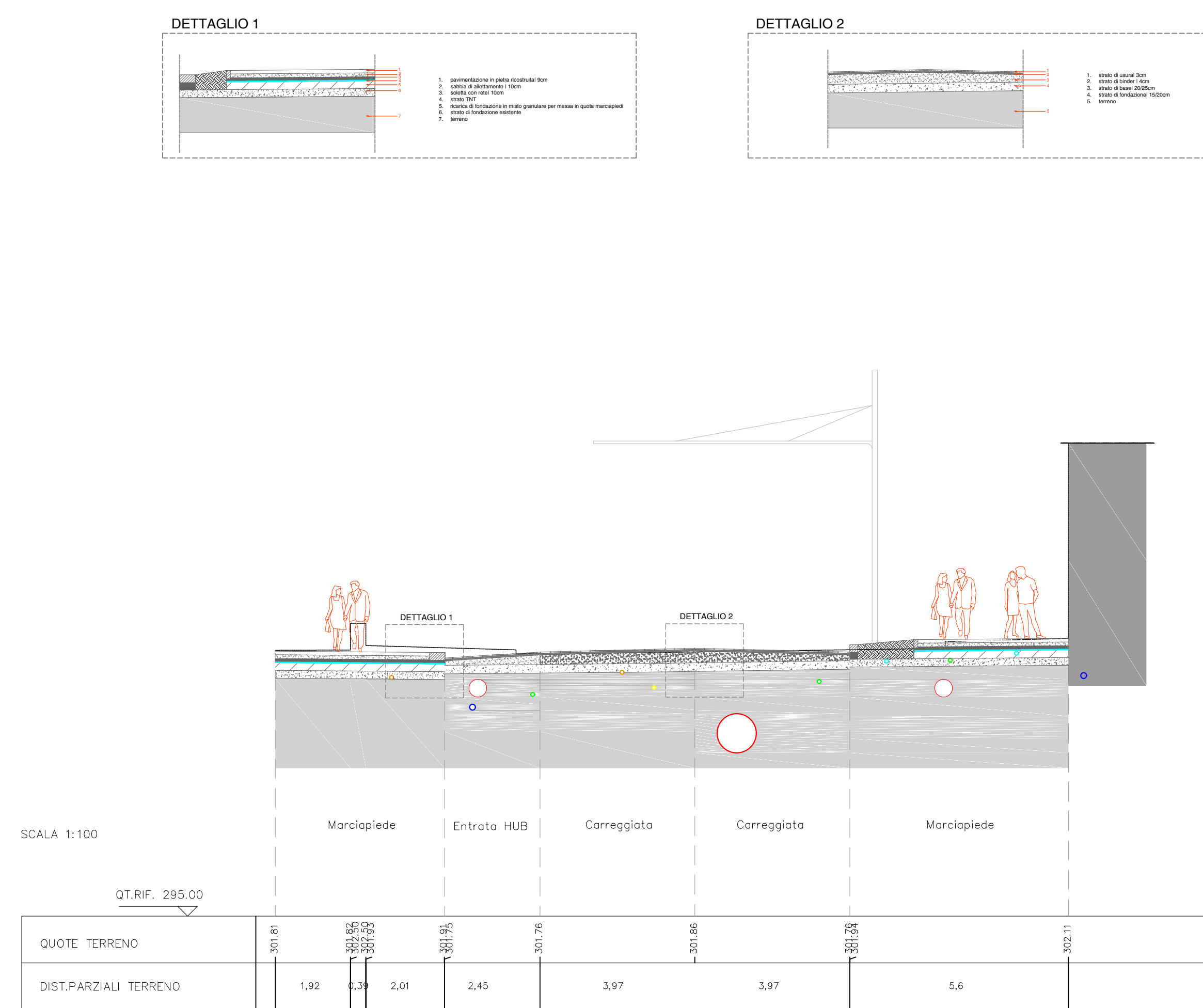
SEZIONE 4_distanza progressiva: 75.00 m
