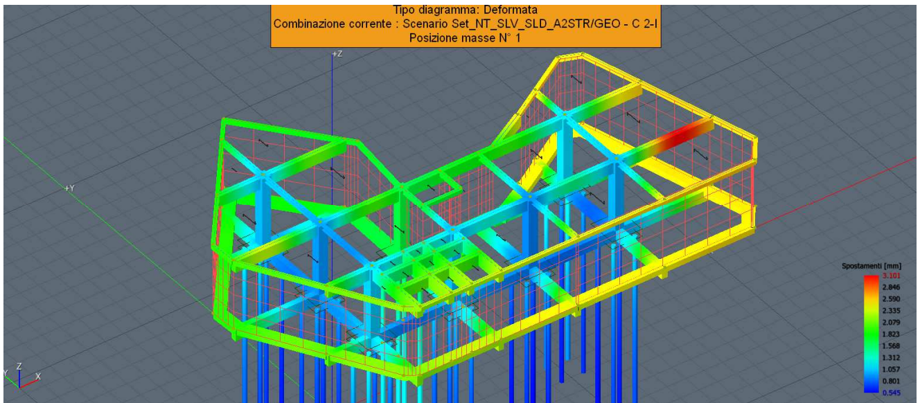
(diagramma tipo dello stato deformativo per carichi verticali)
