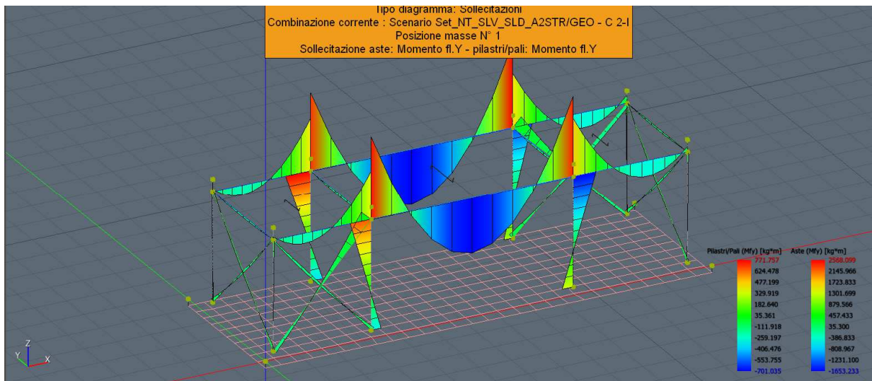
(sollecitazione telai in elevazione – momento flettente – carichi verticali)
