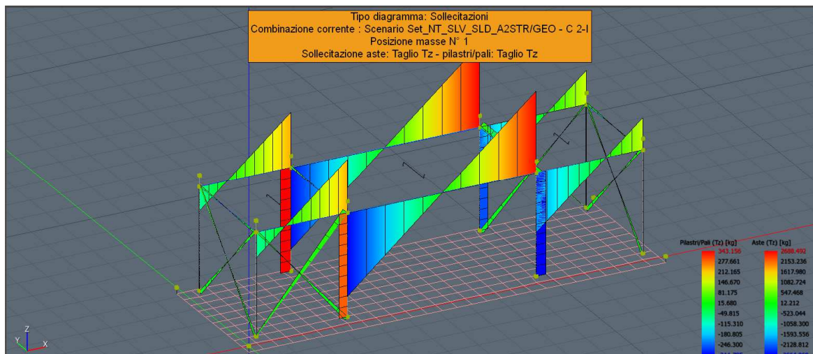
(sollecitazione telai in elevazione – taglio – carichi verticali)
