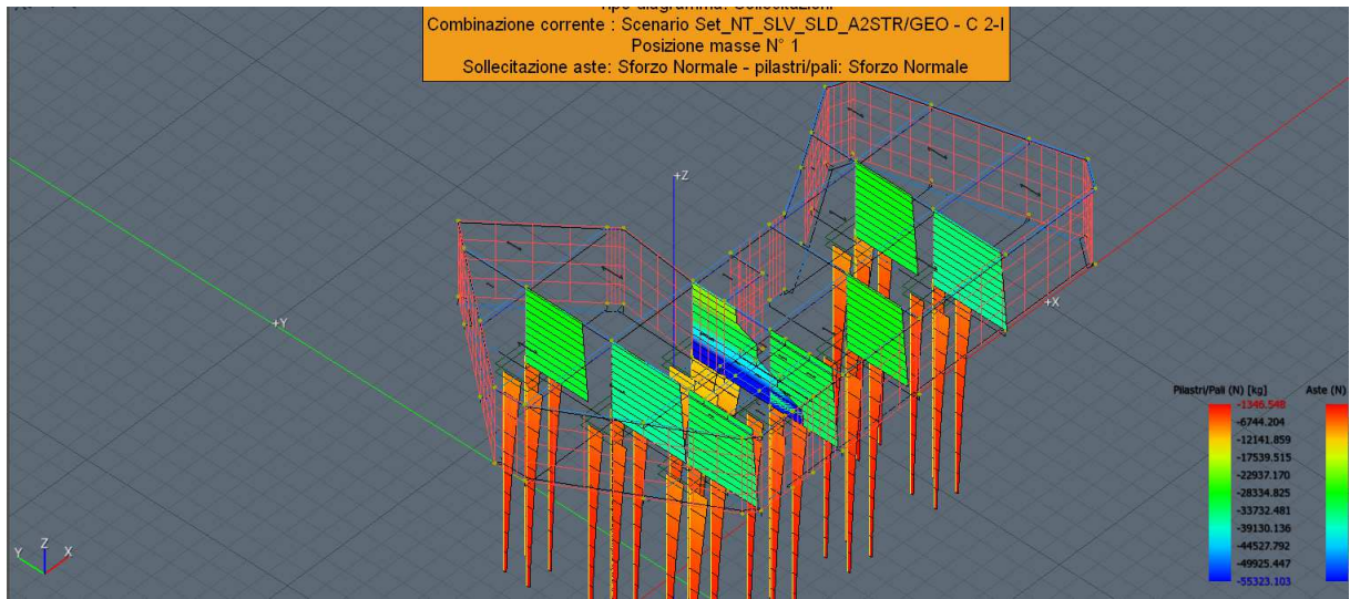
(diagramma tipo delle sollecitazioni da momento flettente)
