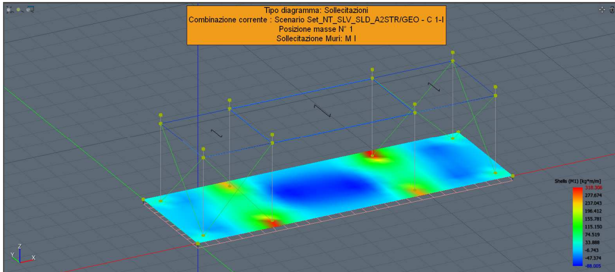
(sollecitazione platea di fondazione)
