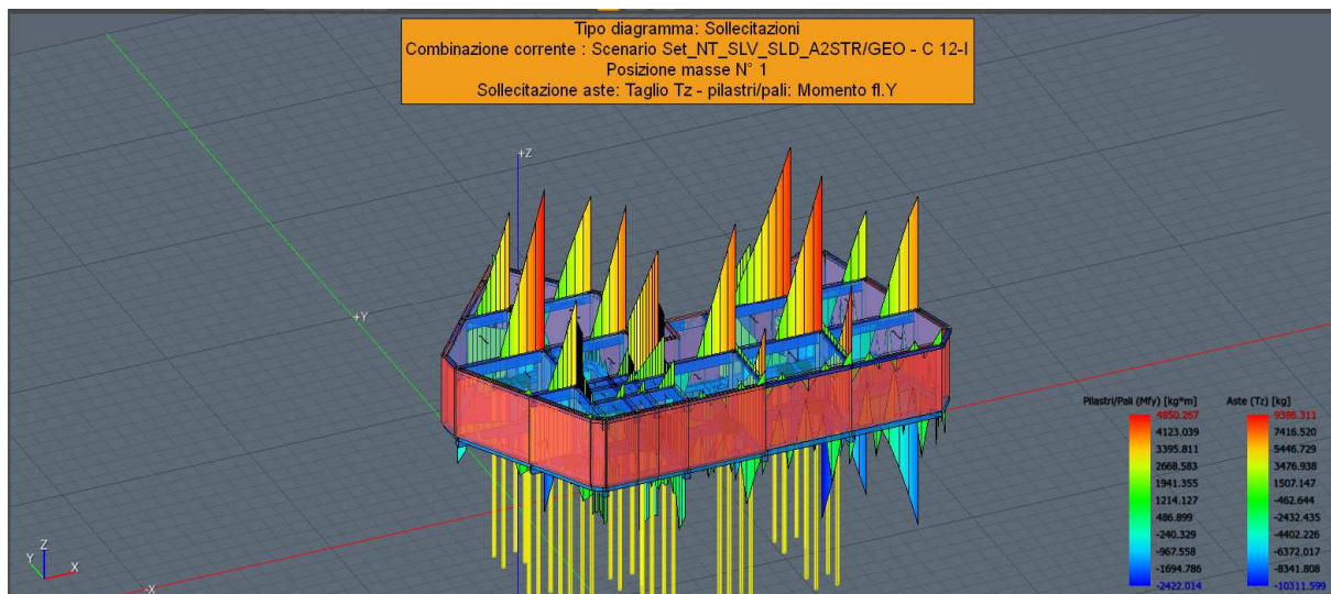
(diagramma tipo delle sollecitazioni da taglio)
