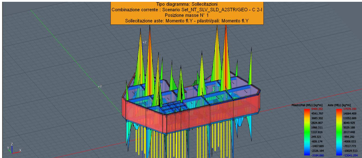
(diagramma tipo delle sollecitazioni da momento flettente)
