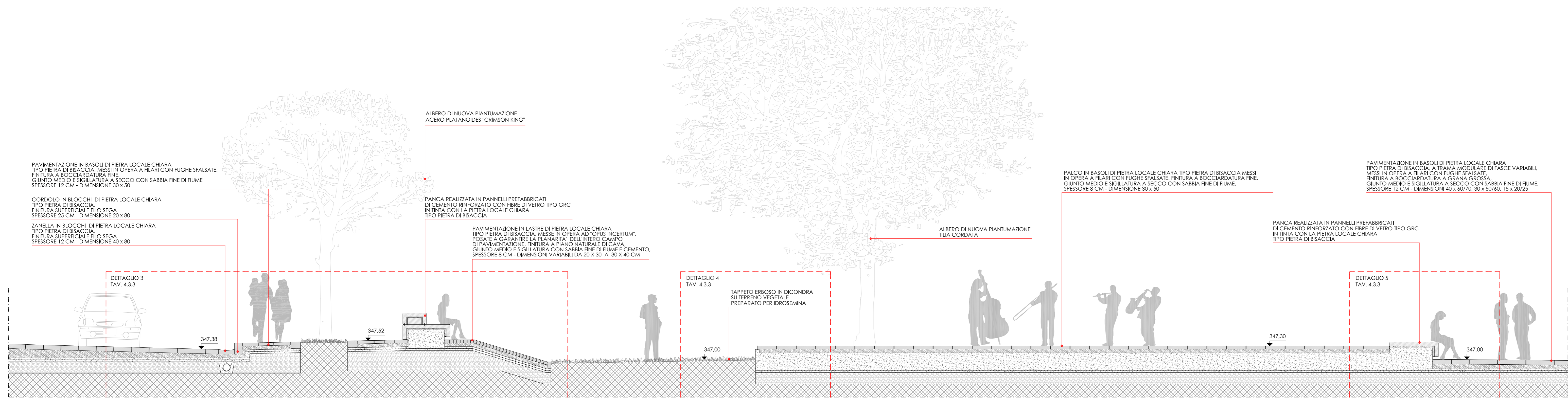
SEZIONE B-B scala 1:50
