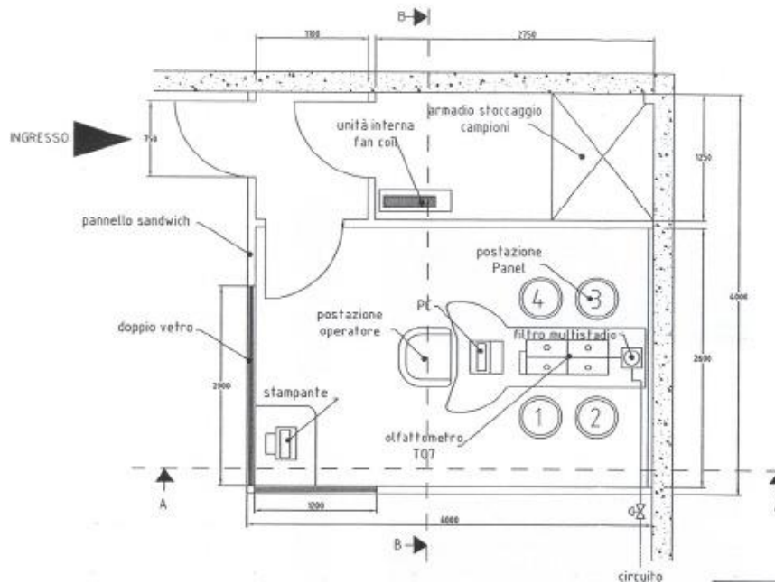
Figura 2: camera olfattometrica.
